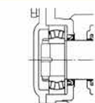
B 轴承详图
