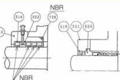
S 轴封详图
