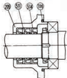
⑤ 轴封详细 轴封详图
