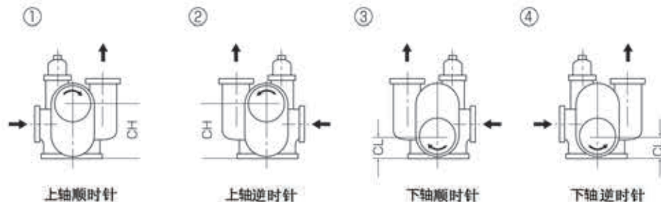
CUL型安装方式和液体流向
